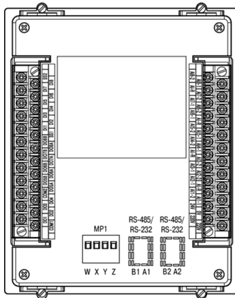
в) задняя стенка корпуса
